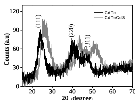
شکل ۱- الگوی پراش اشعه ایکس نقاط کوانتومی کادمیم تلوراید و هسته/پوسته‌ی کادمیم تلوراید/کادمیم سولفید.
