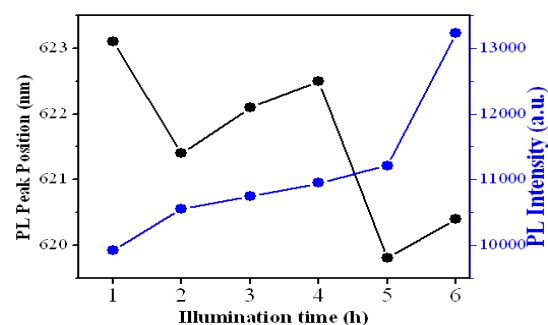
شکل ۳- محل قله و شدت فلئورسانس نقاط کوانتومی هسته-پوسته کادمیم تلوراید-کادمیم سولفید
