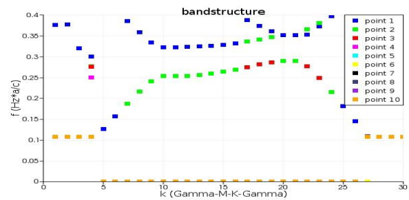
شکل ۱: ساختار نواری تیغه فوتونیک کریستال دو بعدی مثلثی با ضریب شکست 3/34 و دوره تناوب و شعاع حفره به ترتیب 0.46/\mu m و 0.115/\mu m میکرومتر و همچنین دارای باند ممنوعه به مرکز حدود 1.556/\mu m .
