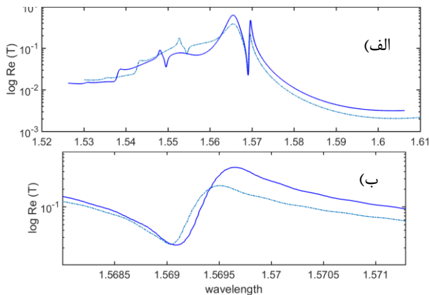
شکل ۴: (الف) طیف فانو خروجی مربوط به ساختار در حالت بهبود کاواک ۱ (خط توپر)، و نمودار شیفیت یافته در طول موج در حالت بدون بهبود (نمودار خط چین). (ب) قسمت بزرگنمایی شده مربوط به طیف فانو. (محور عمودی نمودارها لگاریتمی است).
