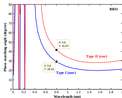
شکل ۱: نمودار جورشدهی فاز بلور BBO جهت تولید SHG [۳و۱].
