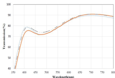
شکل ۲: طیف تراگسیل نمونه‌ها در آهنگ‌های لایه‌نشانی متفاوت
