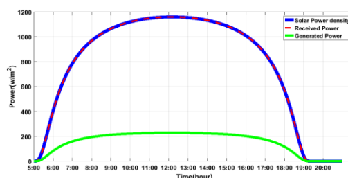
شکل ۶: توان پرتوهای خورشیدی، توان دریافتی و توان تولیدی پنل متحرک برای شهر تهران در تاریخ ۹۶/۰۴/۲۴.
