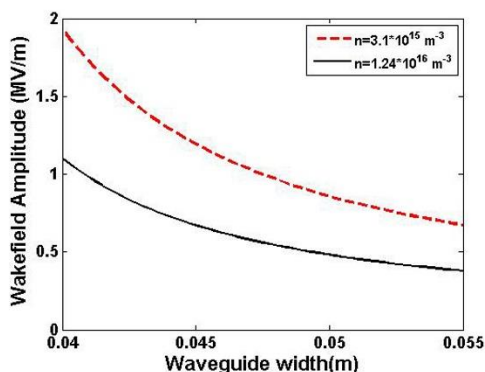
شکل ۶. تغییرات ماکزیمم دامنه میدان دنباله پالس گاوسی بر حسب عرض موجبر برای f = 5 \text{ GHz} , I = 10^{10} \frac{\text{W}}{\text{m}^2}
