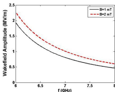
شکل ۵. تغییرات ماکزیمم دامنه میدان دنباله پالس در موجبر مستطیلی بر حسب فرکانس پالس به عرض a = 4 \text{ cm}
