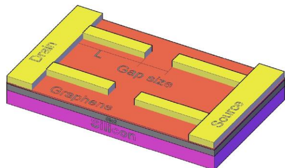
شکل ۴: شماتیک سه بعدی از آشکارساز نوری_گرافنی بهبود داده شده با نانو ذرات فلزی. ساختار در جهت طولی و عرضی متناوب می باشد، دوره ی تناوب نانو ذرات در جهت عرضی 1/2 \mu m می باشد، هر یک از شکاف های ما بین آنتن ها به عنوان یک نانو آشکارساز نوری در نظر گرفته شده است.
