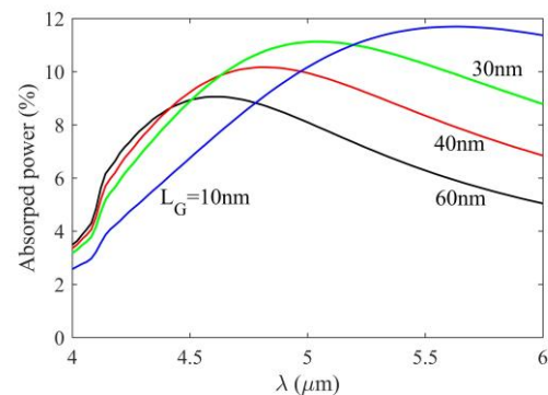
شکل ۴: درصد توان جذب شده در سطح گرافن بر حسب فاصله شکاف بین آنتن ها.
