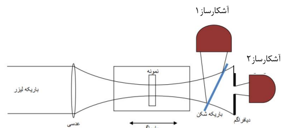
شکل ۱: چیدمان تجربی روبش Z.
