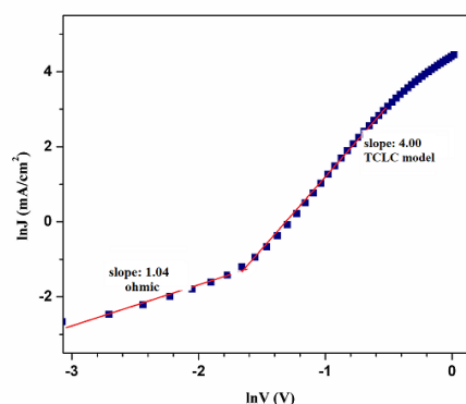
شکل ۵: منحنی مشخصه \ln J - \ln V برای سلول فتوولتاییک پلیمری P3HT:PCBM با نسبت وزنی ۱:۱
