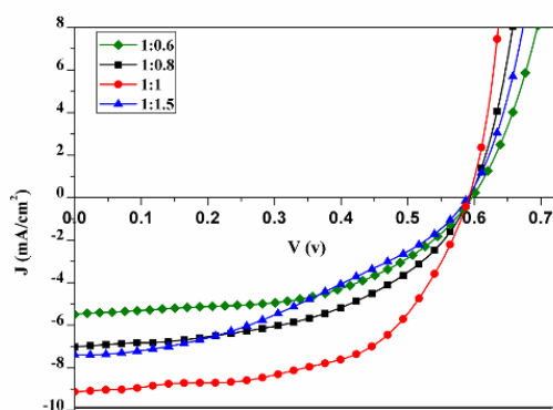
شکل ۳: منحنی مشخصه چگالی جریان-ولتاژ تحت روشنایی
