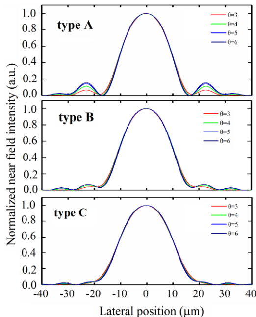
شکل ۲: شدت میدان نزدیک بر حسب مکان در جهت جانبی در لیزر دیوهای مخروطی نوع A (دایره)، نوع B (وسط) و نوع C (پایین) با R_f=0.05 ، W_{\text{ridge}}=3\mu\text{m} و توان خروجی ۱ وات
