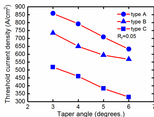
شکل ۵: چگالی جریان آستانه بر حسب زاویه قسمت مخروطی در لیزر دیوهای مخروطی نوع A (دایره)، نوع B (مثلث) و نوع C (مربع) با R_f=0.05 , W_{ridge}=3\mu m
