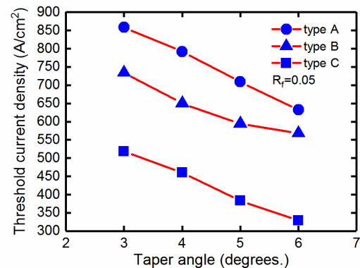
شکل ۵: چگالی جریان آستانه بر حسب زاویه قسمت مخروطی در لیزر دیوهای مخروطی نوع A (دایره)، نوع B (مثلث) و نوع C (مربع) با R_f=0.05 , W_{ridge}=3\mu m
