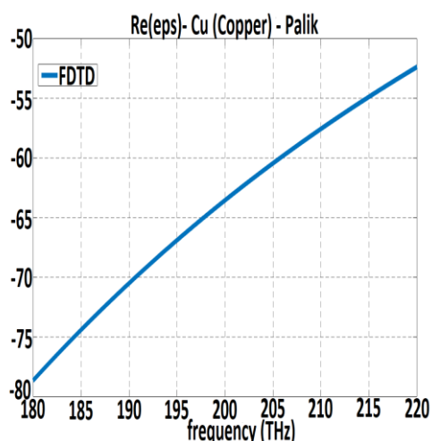
شکل ۶: قسمت حقیقی ضریب دی الکتریک مس از داده های Palik.
