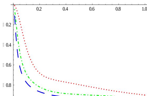
شکل ۲: نمودار پارامتر مندل برحسب Z به ازای N=2 (نقطه چین) و N=4 (خط نقطه چین) و N=6 (خط چین).
