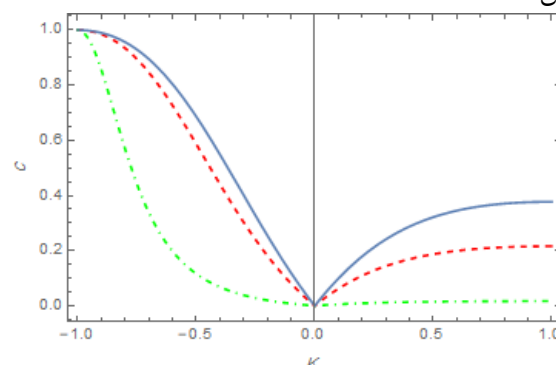
شکل ۲: ضریب توافق برحسب تابعی از k ، به ازای n = 10 و m = 3 و m = 12 (منحنی خط-نقطه) و m = 20 (منحنی توپر).
