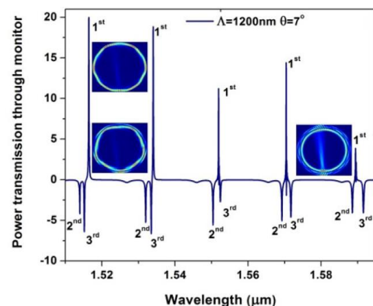
شکل ۵: توان عبوری از مانیتور بر حسب طول موج در جفت‌شدگی عمودی که با تحریک ۳ مرتبه از مدهای شعاعی همراه است [۷].
