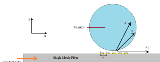
شکل ۱: نمایش دوبعدی جفت‌شدگی نور در حالت توری-جانبی
