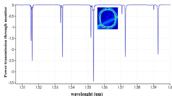
شکل ۲: نمودار توان عبوری از مانیتور تعبیه شده نزدیک سطح میکرودیسک بر حسب طول موج در حالت توری-جانبی
