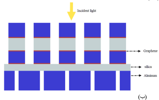
شکل ۱: (الف) نمای سه بعدی قطبشگر مبتنی بر گرافن (ب) نمای دو بعدی قطبشگر مبتنی بر گرافن
