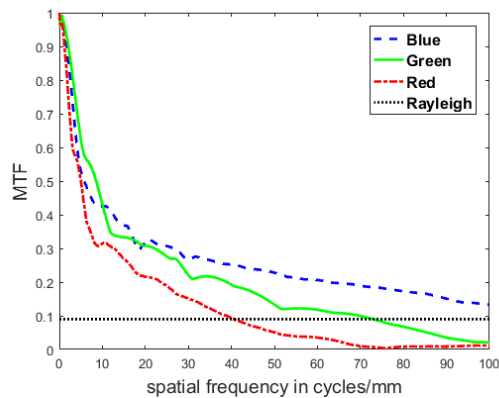
شکل ۶: نمودار MTF موثر در روش پوشش طیفی برای لنز آکرومات نمونه و زاویه ۱۰ درجه.
