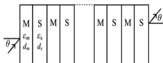
شکل ۴: نانوبلور فوتونی ابررسانا شامل فراماده (M-S)^N
