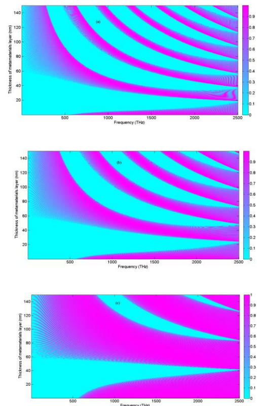
شکل ۴: تاثیر ضریب گذردهی فراماده در طیف تراگسیل نانوبلور فوتونی ابررسانا شامل فراماده (M-S)^N بر حسب ضخامت فراماده الف) \epsilon_m = -10 (ب) \epsilon_m = -6 و ج) \epsilon_m = -2
