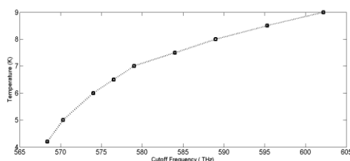
شکل ۵: تاثیر دمای اعمالی در فرکانس قطع نانوبلور فوتونی
