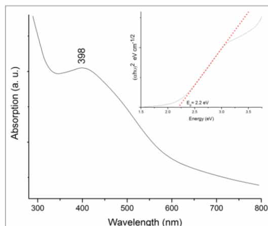
شکل ۲: طیف جذب UV-Vis نمونه و منحنی (\alpha h\nu)^2 بر حسب h\nu
