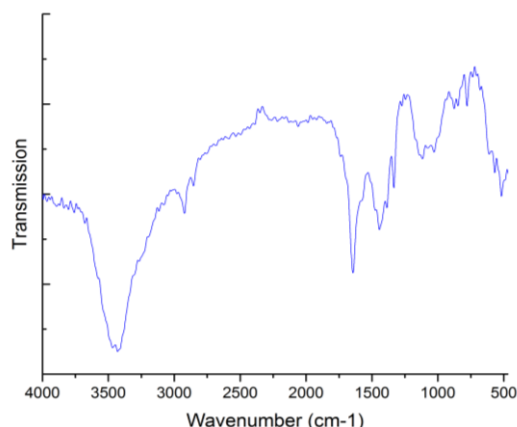
شکل ۴: طیف FTIR به دست آمده از نانوذرات سنتز شده در ناحیه طیفی ۴۰۰۰-۴۰۰
