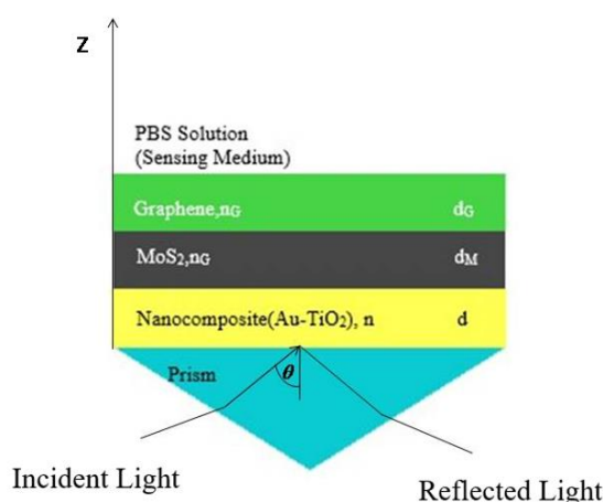
شکل ۱: تصویر شماتیک از ساختار پیشنهادی بیوسنسور نوری مبتنی بر تشدید پلاسمون سطحی حاوی لایه های نانوکامپوزیت، MoS 2 و گرافن.
