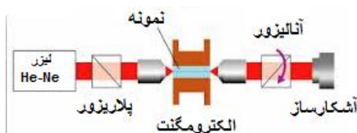
شکل ۱: چیدمان اثر مگنتوپتیکی فاراده.
