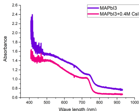
شکل ۴: تغییرات جذب بر حسب طول موج در دو حالت با سزیم و بدون سزیم
