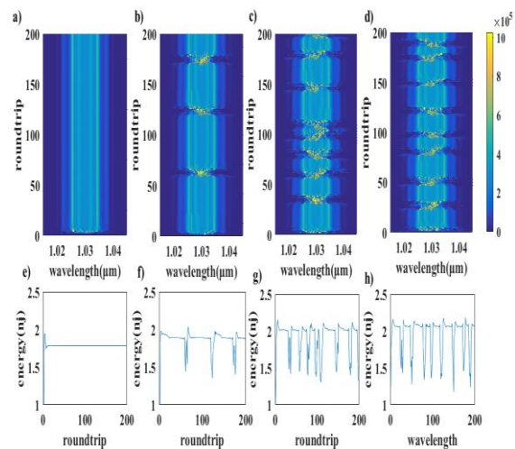
شکل ۴: تحول شکل طیفی و انرژی پالس خروجی به ازای توانهای
