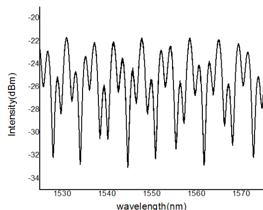
شکل ۲: طیف تداخلی بازتابی حسگر پلیمری
