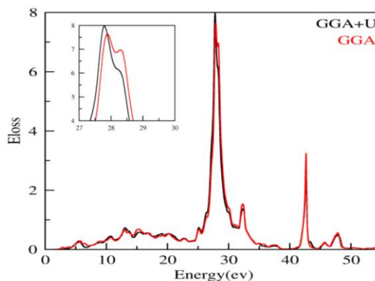
شکل ۳: نمودار تابع اتلاف انرژی ترکیب \text{Sr}_2\text{NiWO}_6
