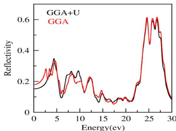
شکل ۴: نمودار ضریب بازتاب ترکیب \text{Sr}_2\text{NiWO}_6
