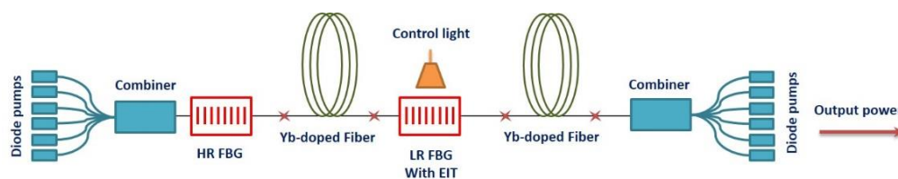
شکل ۱: نمای از MOFPA بر مبنای FBG-EIT ۱۵۸
