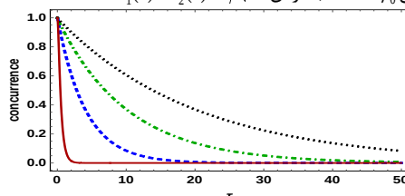
شکل ۱: کمیت تلاقی برحسب \tau = \gamma_0 t در محیط مشترک برای بسامدهای رابی متفاوت به ازای \Delta = 0 (شکل بالا) و به ازای \Delta = \gamma_0 (شکل پایین). \Omega = 0 (خط پیوسته)، \Omega = 0.1\gamma_0 (خط چین)، \Omega = \gamma_0 (نقطه-خط) و \Omega = 3\gamma_0 (نقطه-چین) در یک محیط غیر-مارکوفی \lambda = 0.1\gamma_0 با فرض c_1(0) = c_2(0) = 1/\sqrt{2} .
