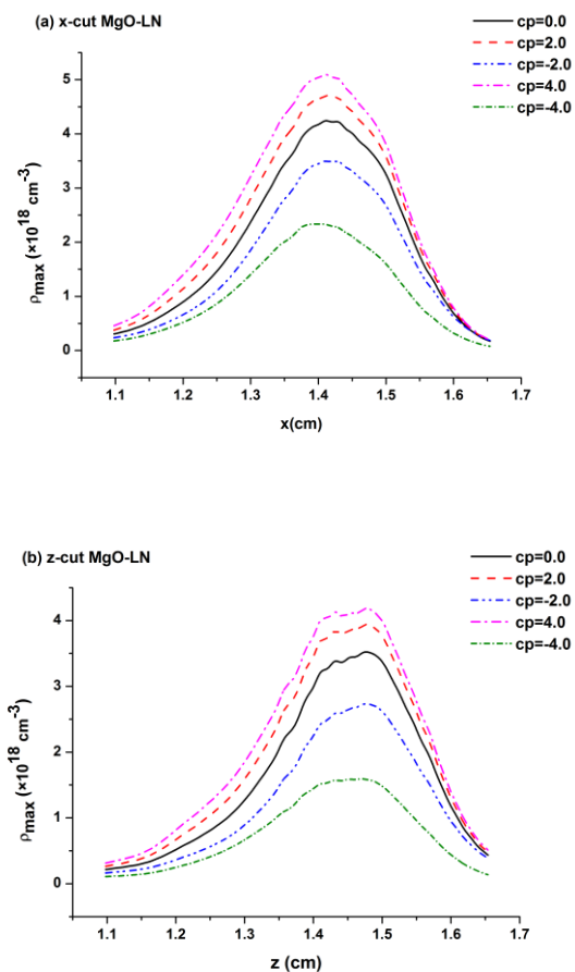
شکل ۲: تغییرات توزیع چگالی پلاسما در محور انتشار به ازای پالسهای لیزری فمتوثانیه با مقدار چیرپ فرکانسی مختلف و با انرژی ۵ میکروژول و طول پالس ۲۵۰ فمتوثانیه کانونی شده داخل کریستال لیتیم نیوبات با (a) برش X و (b) برش Z
