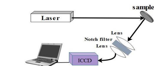
شکل ۱: طرح‌واره چیدمان بیناب‌نمایی رامن
