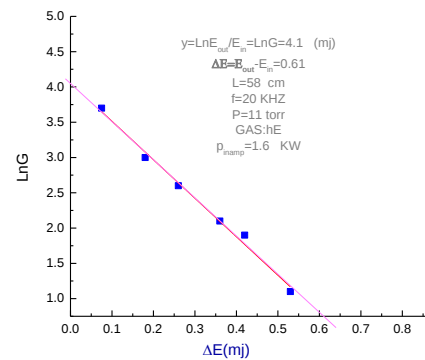
( شکل ۲) نمودار بهره انرژی \ln G بر حسب اختلاف انرژی
