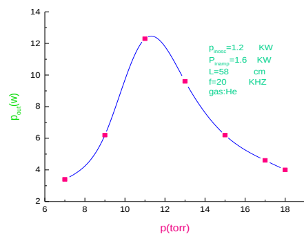
شکل ۵ رفتار توان بر حسب فشار گاز کمکی هلیوم برای تقویت کننده بطول ۵۸cm
