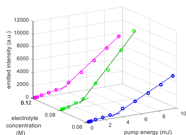
شکل ۵: منحنی شدت قله‌ی تابشی بر حسب انرژی بر پالس پمپ برای نمونه‌های رشد داده شده با غلظت‌های متفاوت ۰/۰۶، ۰/۰۸ و ۰/۱۲ مولار نیترات روی.
