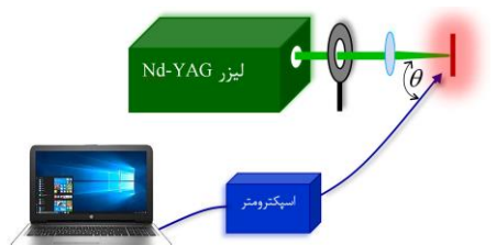
شکل ۲: طرح‌واره‌ای از چیدمان آزمایش.
