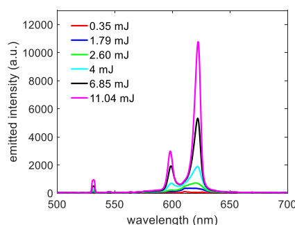
شکل ۳: تغییر طیف تابشی با افزایش انرژی دمش بر حسب میلی ژول بر پالس.
