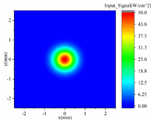
شکل ۲: نیمرخ پرتو سیگنال در ورود به بلور
