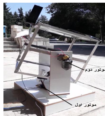
شکل ۲- ساختار مکانیکی ردیاب
