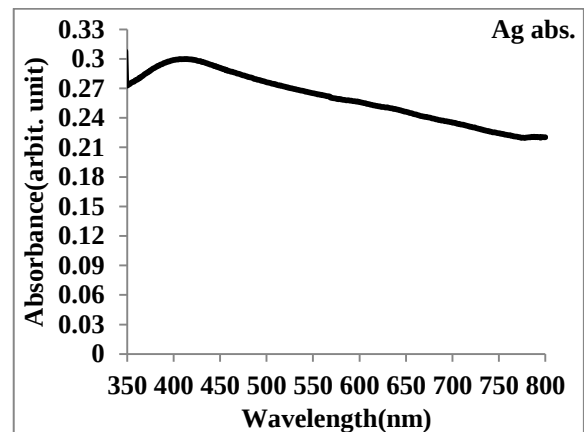
شکل ۴: بیناب جذب نوری محلول نانوذرات نقره.
