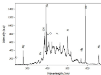
شکل ۲: بیناب LIBS باکتری E.coli
