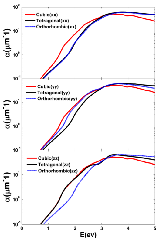
شکل ۱- ضریب جذب بر حسب انرژی در سه فاز مختلف
