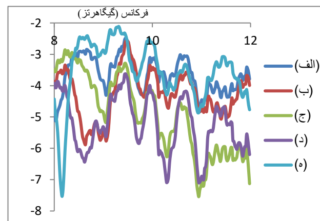
شکل ۸: نمودار اتلاف انعکاس بر حسب فرکانس نمونه ۵-۱.
