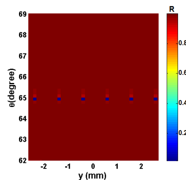
شکل ۵: نمودار بازتابندگی بر حسب تغییرات عرضی y و زاویه تابش. ضریب شکست آنالیت n_{\text{Analyte}} = 1.33 و زاویه تابش 65^\circ درجه انتخاب شده است.
