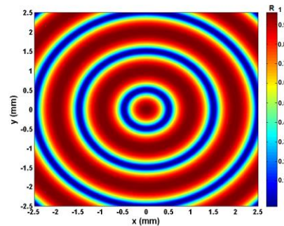
شکل ۴: نمودار بازتابندگی بر حسب تغییرات x و y ، که طول موج نور فرودی \lambda_0 = 632.8 \text{ nm} (لیزر هلیوم-نئون) و ضریب شکست آنالیت n_{\text{Analyte}} = 1.33 و زاویه تابش 65^\circ درجه انتخاب شده است.
