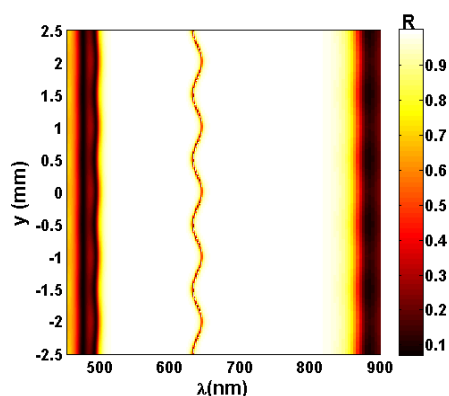
شکل ۳: طیف بازتابی از ساختار بر حسب فاصله عرضی y . ضریب شکست آنالیت n_{Analyte} = 1.33 و زاویه تابش ۶۵ درجه انتخاب شده است.
