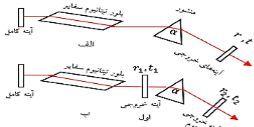
شکل ۱: کاواک لیزر تیتانیوم سفایر: الف) چیدمان درون کاواکی ب) چیدمان بیرون کاواکی
