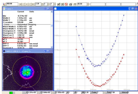
شکل ۸: اندازه‌گیری کیفیت باریکه، برای پرتو خروجی نهایی از فیبر 200\mu\text{m} ، در توان ۵ کیلووات، با استفاده از دستگاه اندازه‌گیری کیفیت پرتو ( M^2 -meter).
