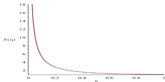
شکل ۲: نمودار اطلاعات فیشر کوانتومی ماتریس چگالی \rho_2 برحسب پارامتر واهمدوسی \eta
