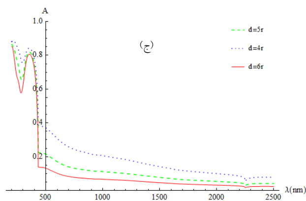
شکل ۱: ضرایب الف عبور، ب انعکاس و ج جذب برحسب طول موج به ازای مقادیر مختلف جدایی ذرات، D = 200nm .
