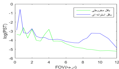
شکل ۳: نمودار لوگاریتم PST بر حسب میدان دید.
