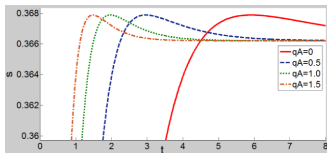
شکل (۲): نمودار آنتروپی بر حسب زمان برای سامانه کیوتریت-کیوتریت تحت کانال نوفه‌ای سه-فیلیپ وقتی q_B = 0.5 (مقدار ثابت) باشد و q_A مقادیر مختلف q_A = 0 (نمودار خط توپر)، q_A = 0.5 (نمودار خط چین)، q_A = 1.0 (نمودار نقطه چین) و q_A = 1.5 (نمودار خط-نقطه چین) را داشته باشد.
