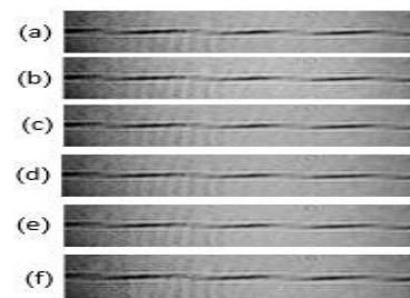
شکل ۳: نقش پراش فرنل از گوه شیشه ای با زاویه گوه
