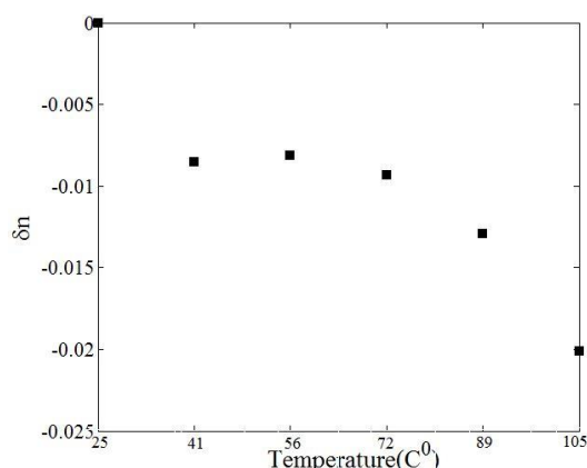
شکل ۵: تغییرات ضریب شکست وابسته به دما بر حسب دما.
