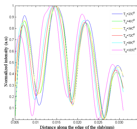
شکل ۴: نمایه شدت فریز مرکزی نقشهای پراش از گوه در دماهای مختلف.
