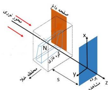
شکل ۲: طرح شماتیک از چیدمان آزمایش
