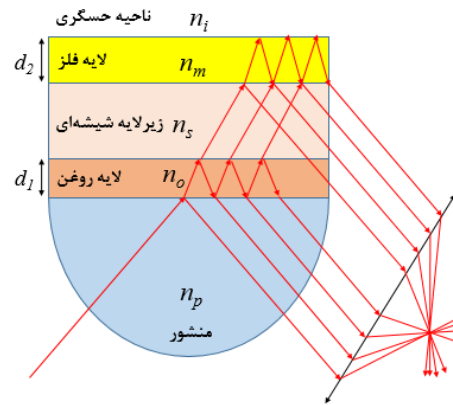
شکل ۳. ساختار حسگر تشدید پلاسمون سطحی
