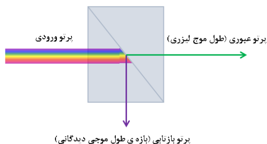
شکل ۱: نمودار طرح‌وار پرتوشکاف مکعبی.
