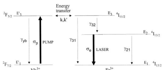
شکل ۱. تراز های انرژی لیزر Er^{+3}:Yb^{+3}:Glass
