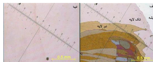
شکل ۵: تصاویر گرفته شده با استفاده از میکروسکوپ نوری. الف: ناحیه‌ای شامل ذرات کلونیدی تک لایه و چند لایه ب: ناحیه‌ای که فقط ذرات کلونیدی تک لایه حضور دارند.
