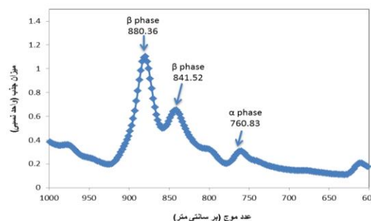
شکل ۴: بیناب FTIR نانوالیاف کامپوزیت PVDF-نانوذرات طلا.
