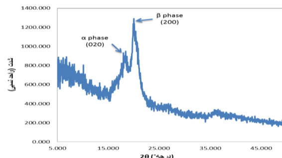
شکل ۳: الگوی XRD نانوالیاف کامپوزیت PVDF-نانوذرات طلا.
